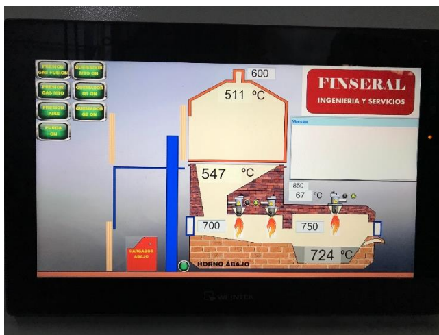
Actual pantalla interface de la torre fusora
